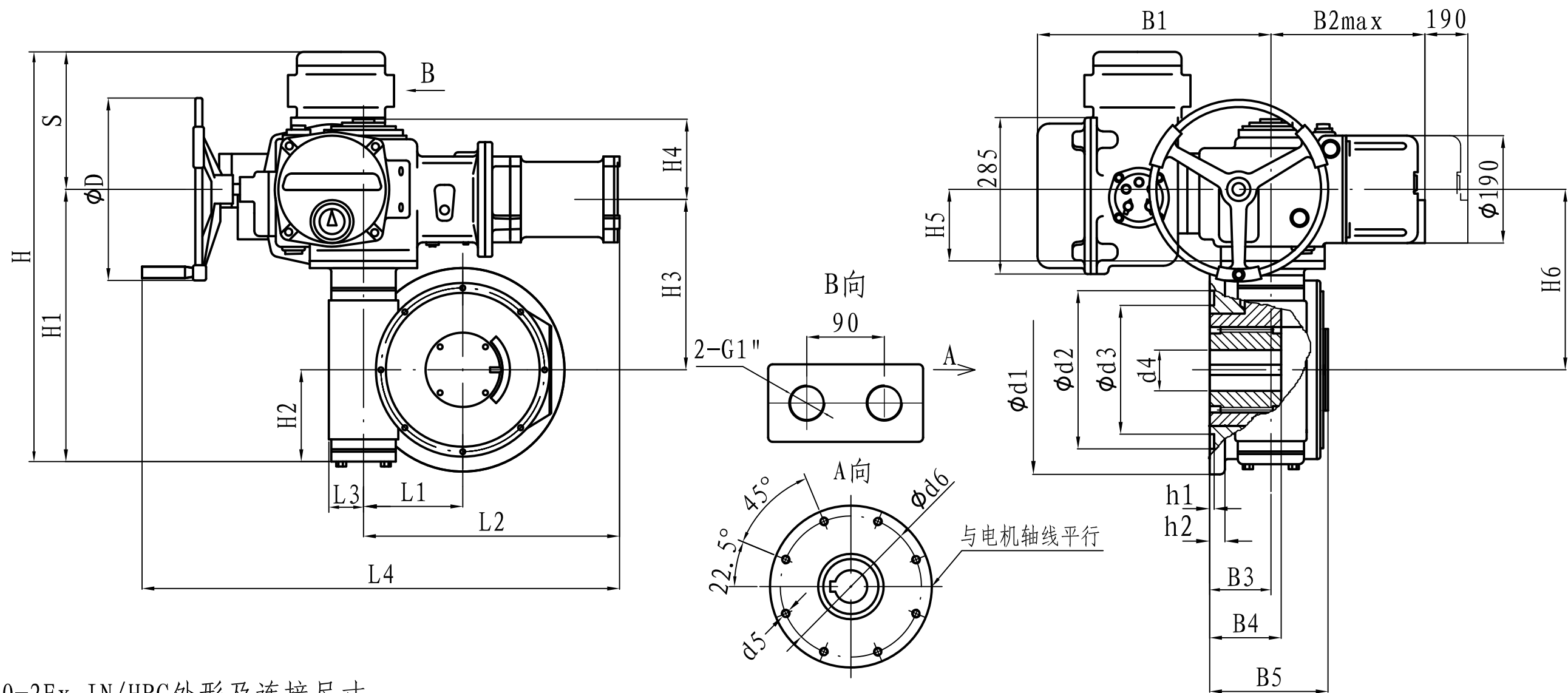
SMC00-2Ex. IN/HBC外形及连接尺寸
